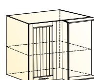
Бавария шкаф навесной угловой (1 дверь глухая) → | 7 | 1 | ↑ 800|400|720
