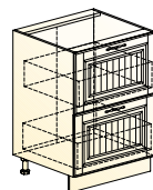
Бавария шкаф рабочий (2 ящика) → | ↗ | ↑ 600|460|820
