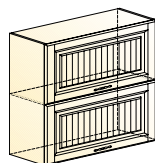
Бавария шкаф навесной (2 двери горизонт.) → | 7 | 1 | ↑ 800|318|720
