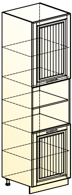
Бавария шкаф-пенал (2 двери) → | ↗ | ↑ 600|570|2141
