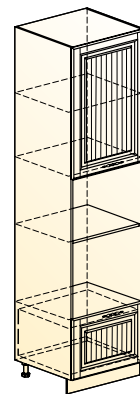
Бавария шкаф-пенал 3 Старт (1 дверь, 1 ящик) → | ↗ | ↑ 600|570|2141
