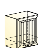
Бавария шкаф навесной под вытяжку (1 дверь глухая) → | 7 | 1 | ↑ 600|318|566
