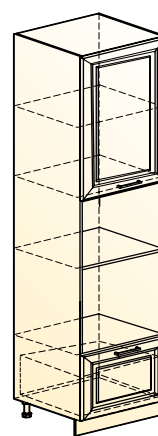
Мишель шкаф- пенал 3 Старт (1 дверь, 1 ящик) → | 7 | ↑ 600|570|2141
