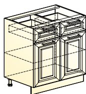
Мишель шкаф рабочий Старт (2 двери 2 ящика) → | 7 | ↑ 800|460|820
