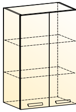
Джаз шкаф навесной (2 двери глухие) → | 7 | | ↑ 600|318|900
