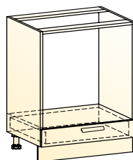
Джаз шкаф рабочий под духовку (1 ящик) → | 7 | 1 | ↑ 600|460|820
