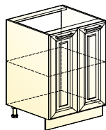
Мишель шкаф рабочий (2 двери) → | 7 | 1 | ↑ 600|460|820
