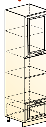
Мишель шкаф- пенал 3 (1 дверь, 1 ящик) → | 7 | ↑ 600|570|2141
