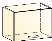
Джаз шкаф навесной (1 дверь глухая) → | 7 | 1 ↑ 500|318|360
