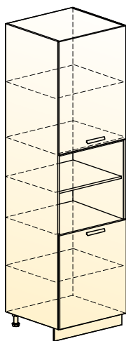
Джаз шкаф-пенал (2 двери) → | 7 | ↑ 600|570|2141
