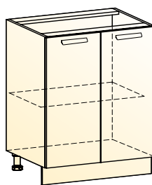
Джаз шкаф рабочий (2 двери) → | 7 | ↑ 600|460|820
