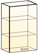
Джаз шкаф навесной (1 дверь глухая) → | 7 | | ↑ 600|318|900
