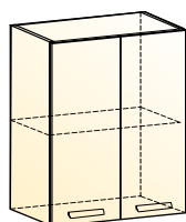
Джаз шкаф навесной (2 двери глухие) → | 7 | 1 ↑ 600|318|720
