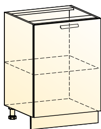
Джаз шкаф рабочий (1 дверь) → | 7 | ↑ 500|460|820
