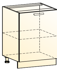
Джаз шкаф рабочий (1 дверь) → | 7 | ↑ 600|460|820
