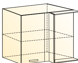
Джаз шкаф навесной угловой (1 дверь глухая) → | 7 | 1 ↑ 800|400|720
