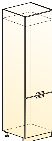
Джаз шкаф-пенал под холодильник (2 двери) → | 7 | ↑ 600|570|2141
