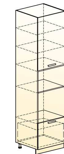
Джаз шкаф-пенал 3 (1 дверь, 1 ящик) → | 7 | ↑ 600|570|2321
