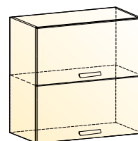
Джаз шкаф навесной (2 двери горизонт.) → | 7 | 1 ↑ 800|318|720
