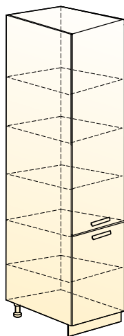
Джаз шкаф-пенал 2 (2 двери) → | 7 | ↑ 400|570|2141
