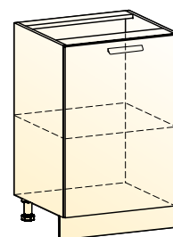
Джаз шкаф рабочий (1 дверь) → | 7 | ↑ 450|460|820
