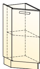
Джаз шкаф рабочий концевой 45° (1 дверь) → | 7 | ↑ 300|564|820
