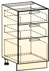
Джаз шкаф рабочий Старт (3 ящика) → | 7 | 1 | ↑ 400|460|820
