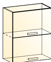
Джаз шкаф навесной (2 двери горизонт.) → | 7 | 1 ↑ 600|318|720
