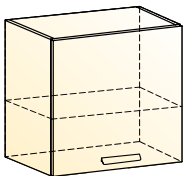
Джаз шкаф навесной (1 дверь глухая) → | 7 | | ↑ 500|318|450
