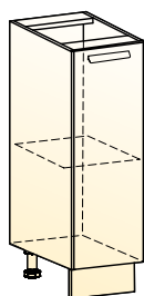
Джаз шкаф рабочий (1 дверь) → | 7 | ↑ 150|460|820
