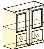
Мишель шкаф навесной (2 двери окошко) → | 7 | 1 | ↑ 800|318|720
