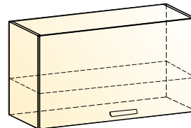
Джаз шкаф навесной (1 дверь глухая) → | 7 | | ↑ 800|318|450
