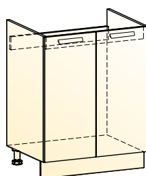
Джаз шкаф рабочий под мойку (2 двери) → | 7 | ↑ 600|456|820
