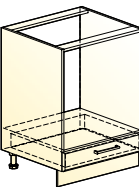
Мишель шкаф рабочий под духовку (1 ящик) → | 7 | ↑ 600|460|820
