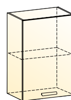
Джаз шкаф навесной (1 дверь глухая) → | 7 | 1 ↑ 500|318|720
