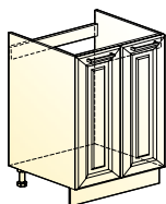
Мишель шкаф рабочий под мойку (2 двери) → | 7 | 1 | ↑ 600|456|820
